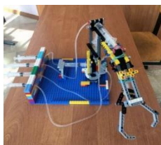
Рис. 1. Гидравлический манипулятор из Lego
