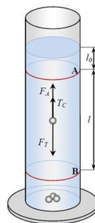
Рис. 3. Лабораторная установка
