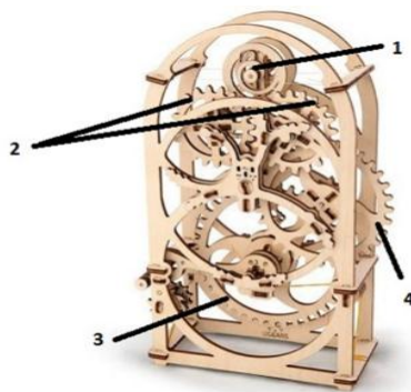
Рис. 1. Собранная модель таймера-секундомера
