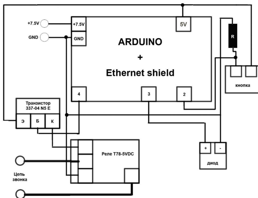
Схема 1. Подключение устройства к цепи звонка
